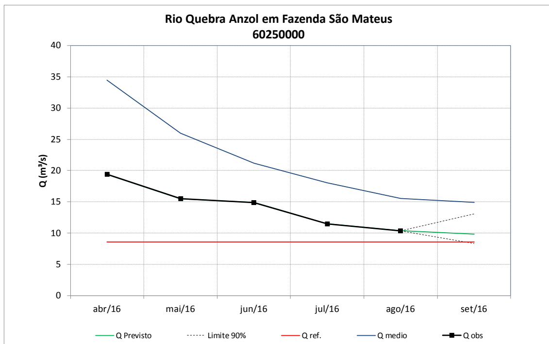
Figura 84 – Previsão de vazões médias do rio Quebra Anzol em Fazenda São Mateus.
