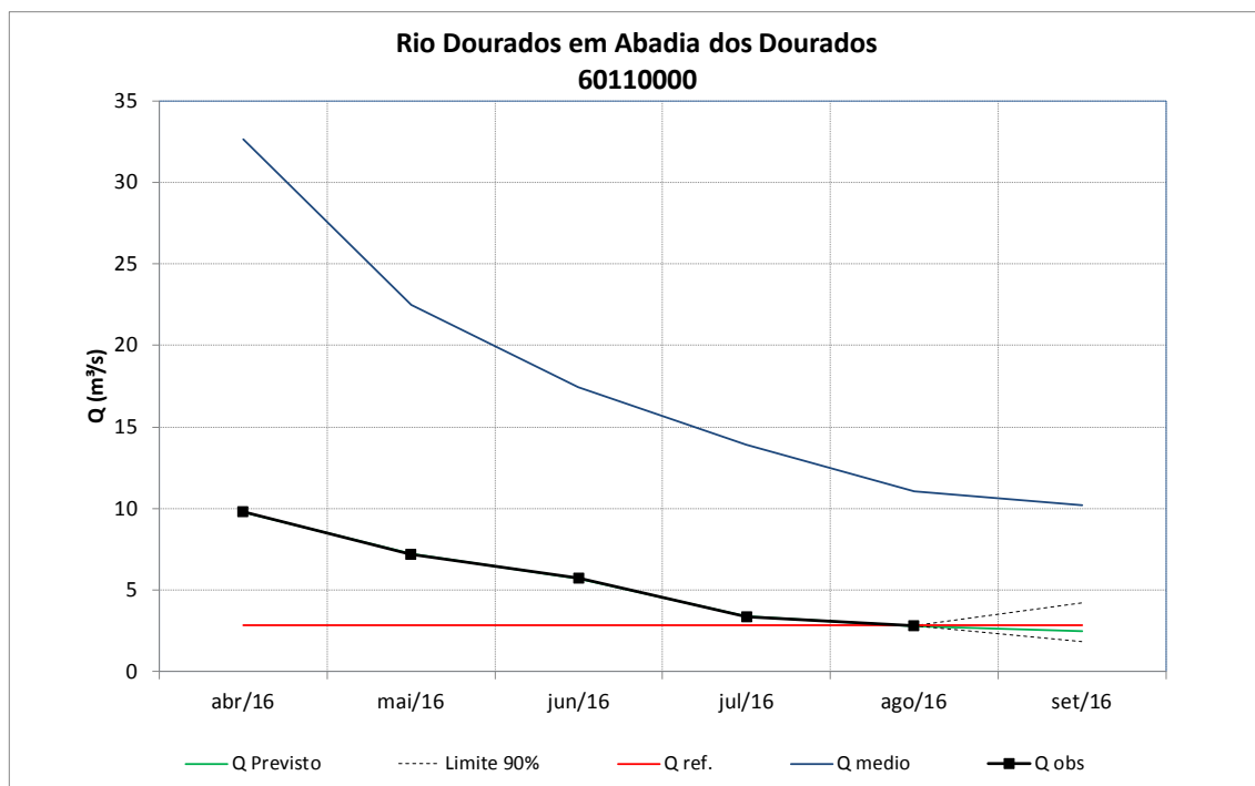
Figura 83 – Previsão de vazões médias do rio Dourados em Abadia dos Dourados.
