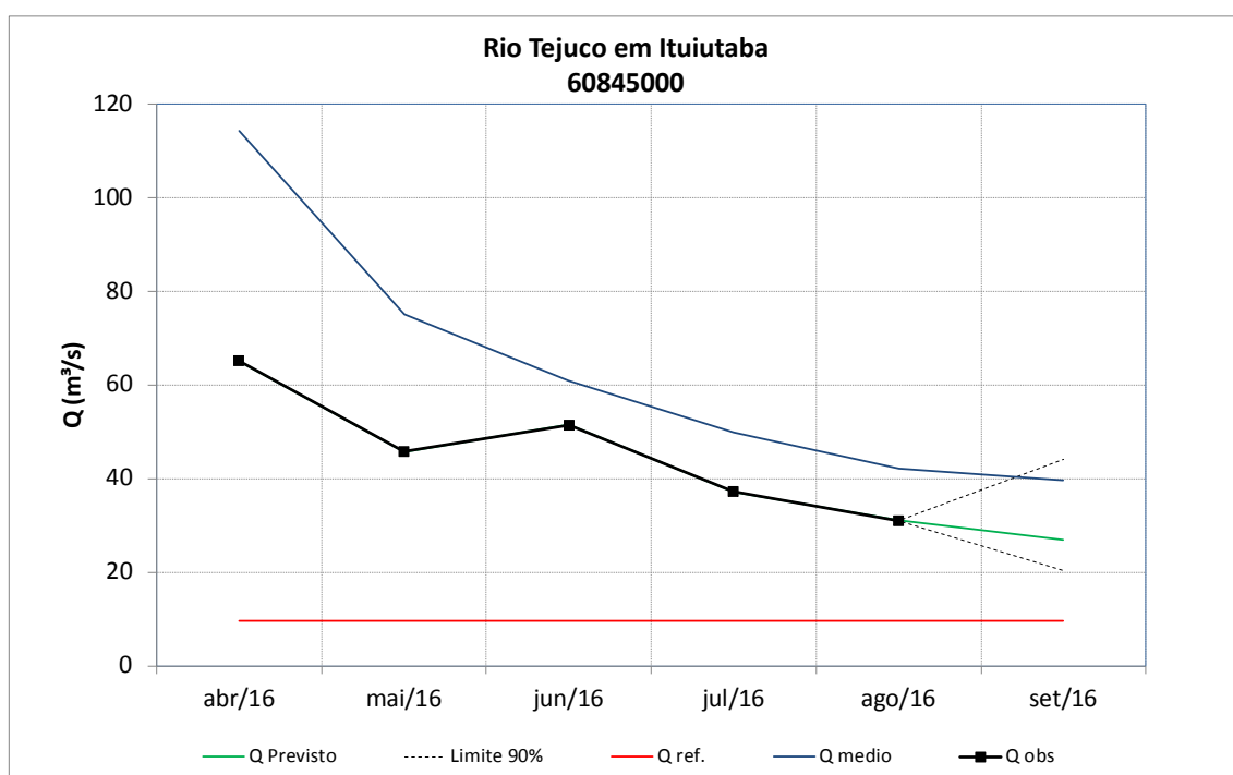
Figura 85 – Previsão de vazões médias do rio Tejuco em Ituiutaba.
