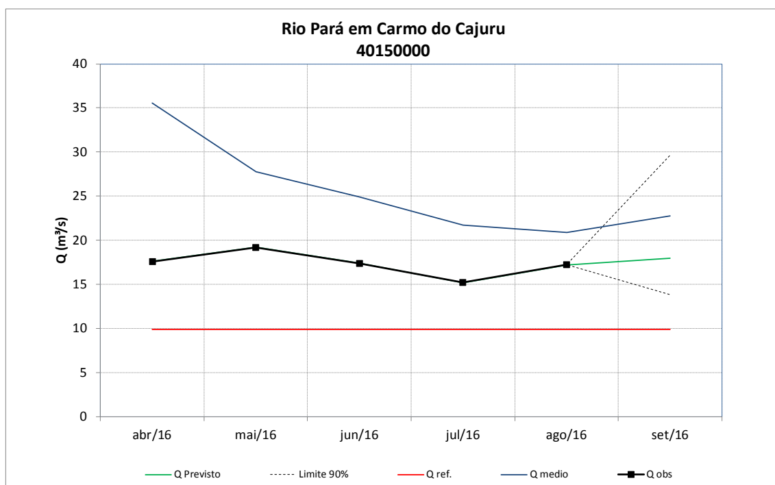
Figura 57 - Previsão de vazões médias do rio Pará em Carmo do Cajuru
