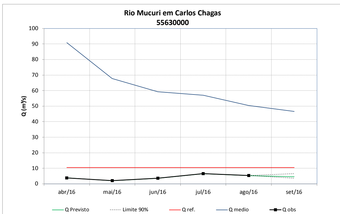
Figura 73 - Previsão de vazões médias do rio Mucuri em Carlos Chagas.
