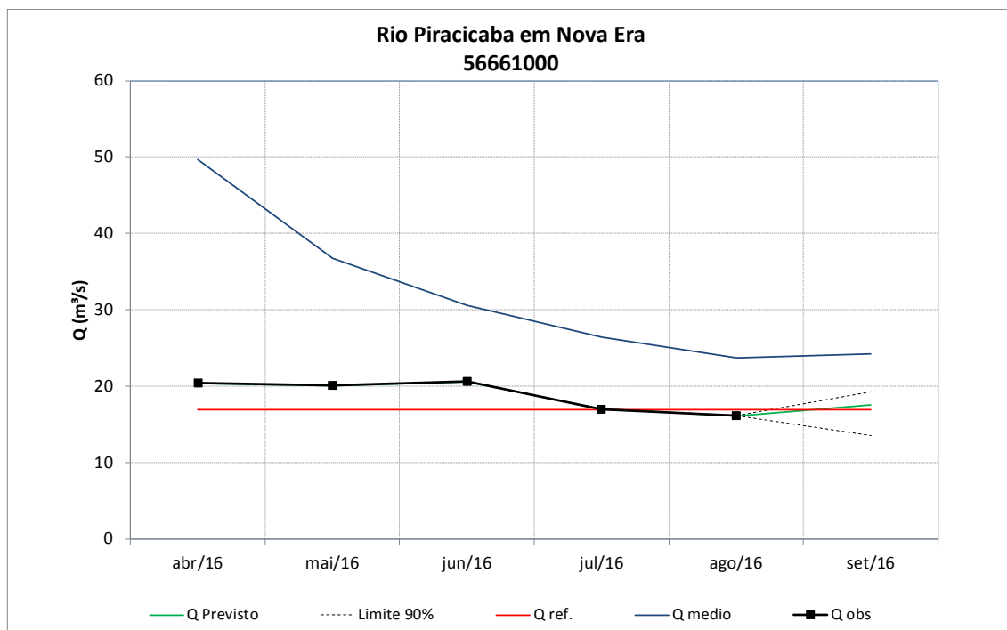
Figura 76 - Previsão de vazões médias do rio Piracicaba em Nova Era.
