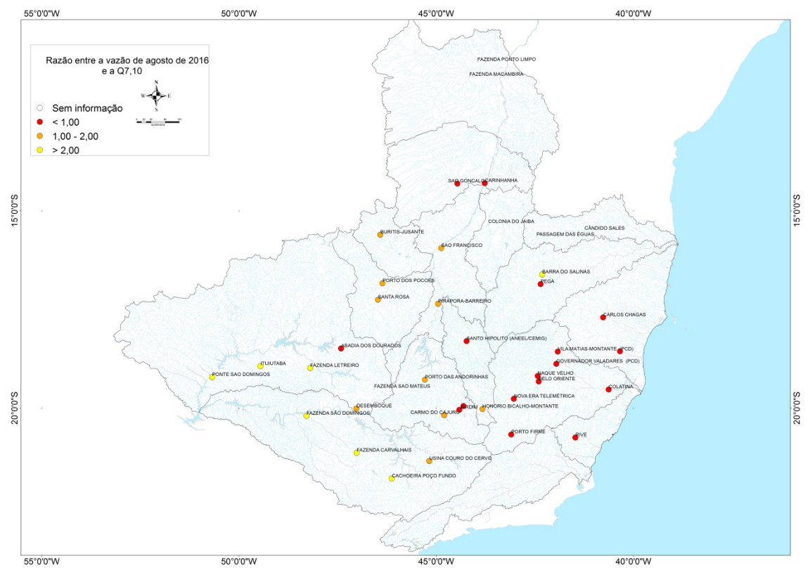
Figura 13 – Razão entre a vazão de agosto de 2016 e a vazão Q 7,10 .
