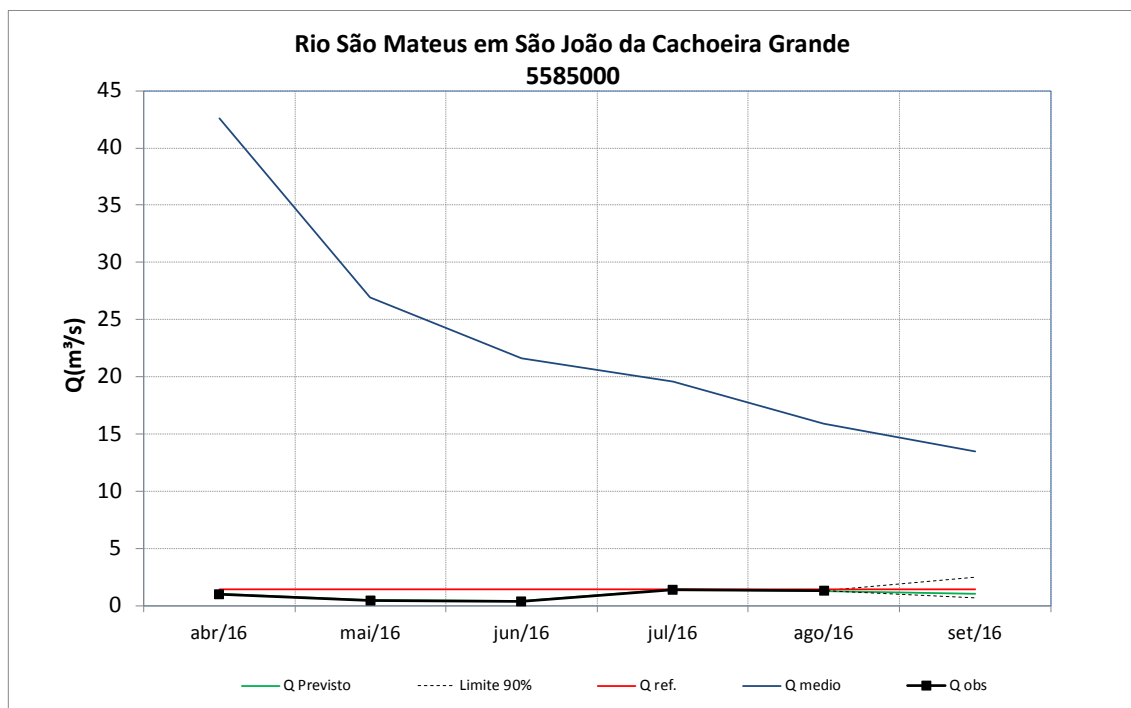
Figura 74 – Previsão de vazões médias do rio São Mateus em São João da Cachoeira Grande.
