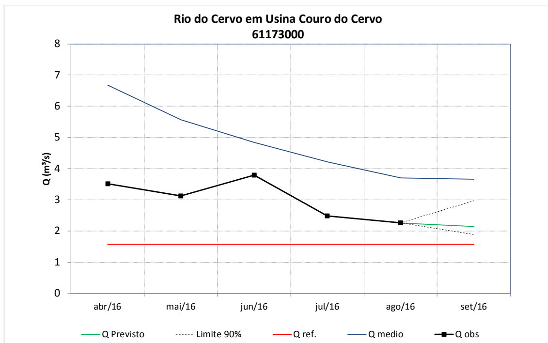
Figura 86 – Previsão de vazões médias do rio do Cervo em Usina Couro do Cervo.
