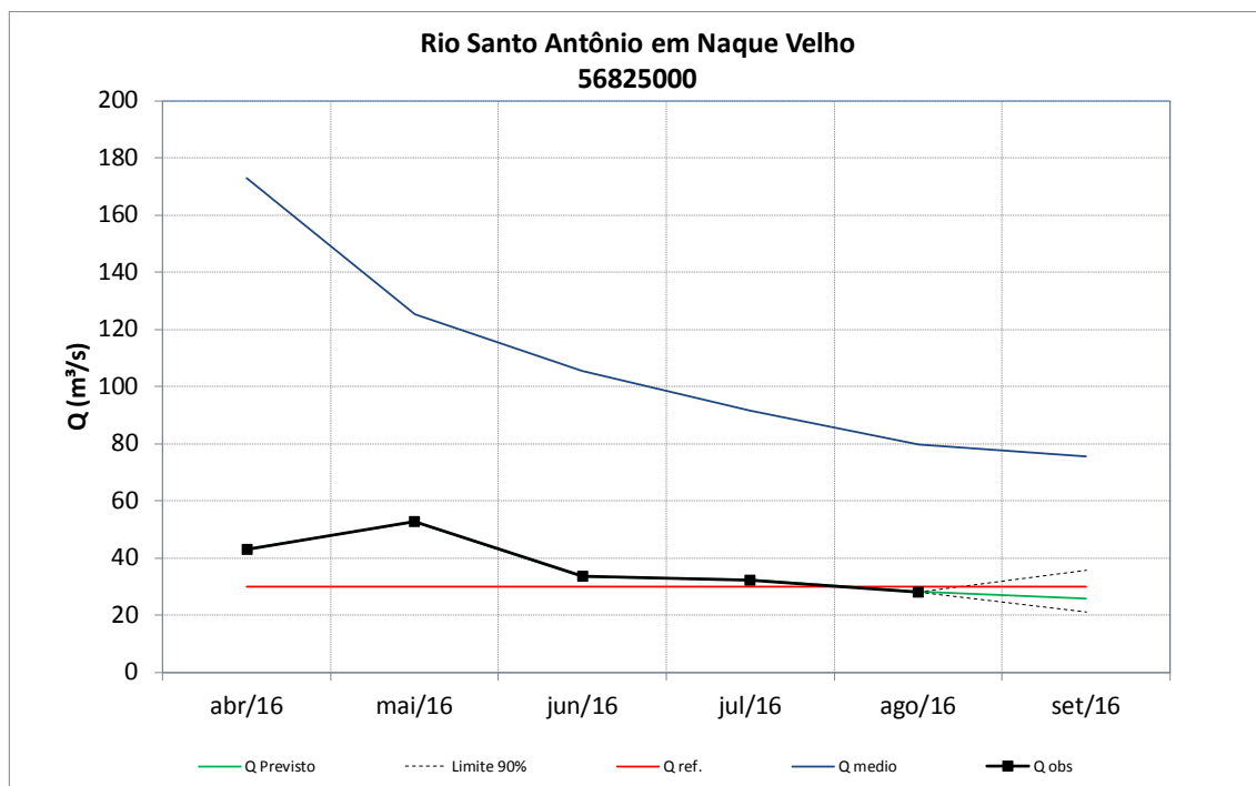
Figura 78 – Previsão de vazões médias do rio Santo Antônio em Naque Velho.
