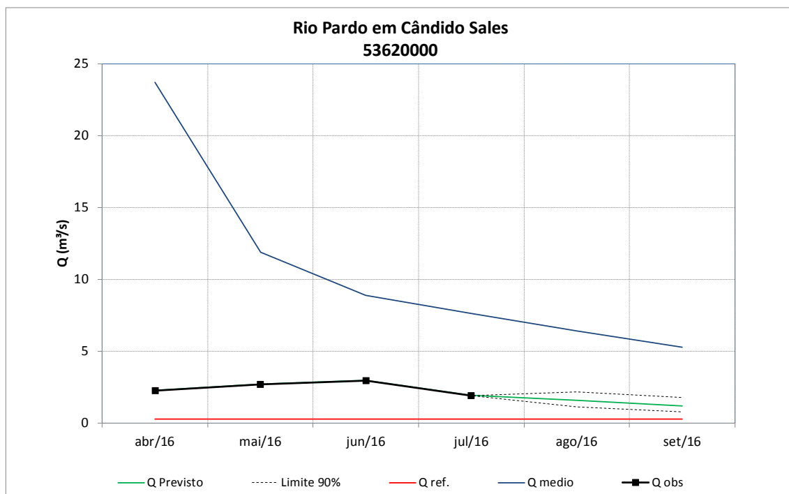
Figura 71 – Previsão de vazões médias do rio Pardo em Cândido Sales.
