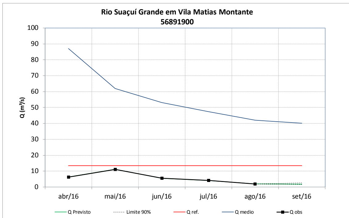
Figura 80 – Previsão de vazões médias do rio Suaçuí Grande em Vila Matias Montante.
