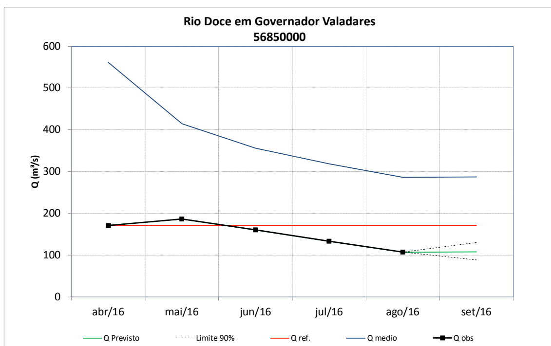
Figura 79 – Previsão de vazões médias do rio Doce em Governador Valadares.
