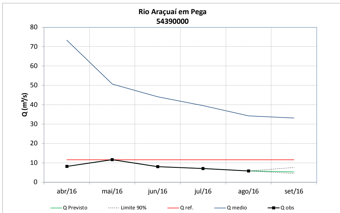
Figura 72 – Previsão de vazões médias do rio Araçuaí em Pega.
