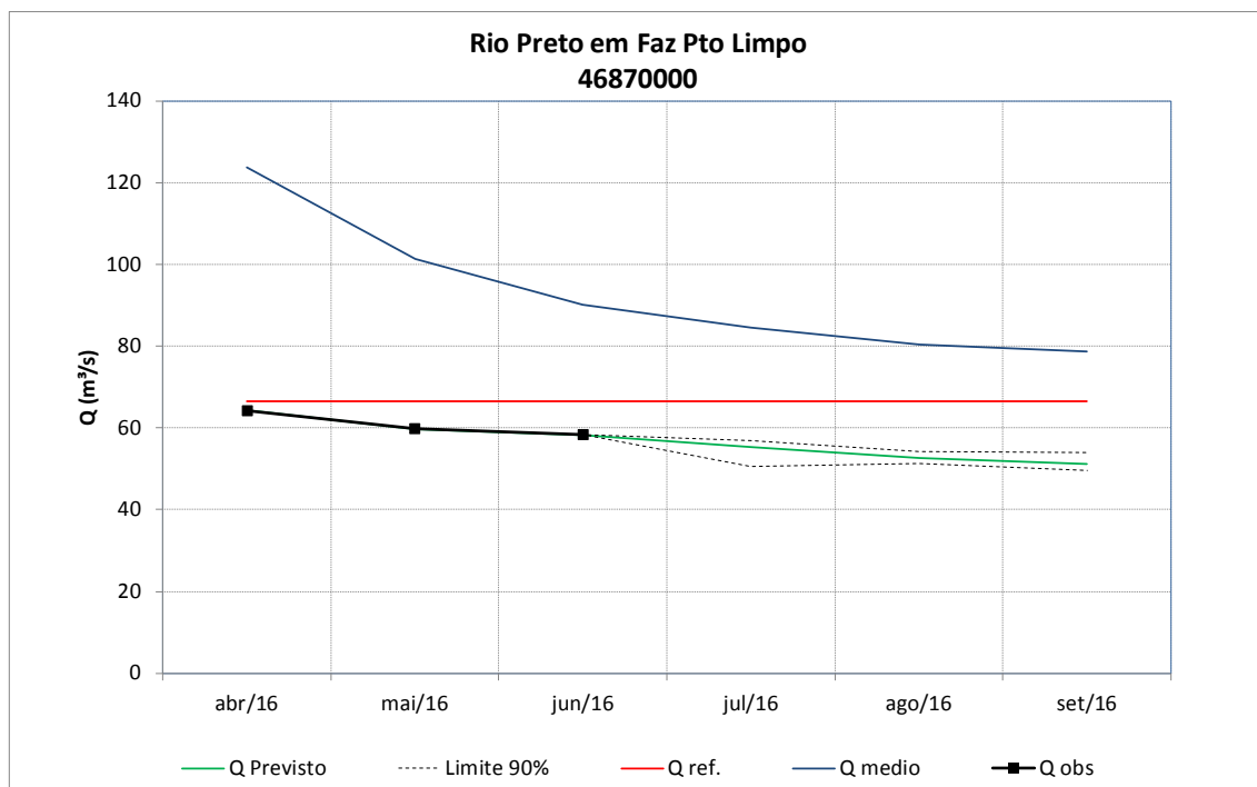
Figura 70 - Previsão de vazões médias do rio Preto em Fazenda Porto Limpo.
