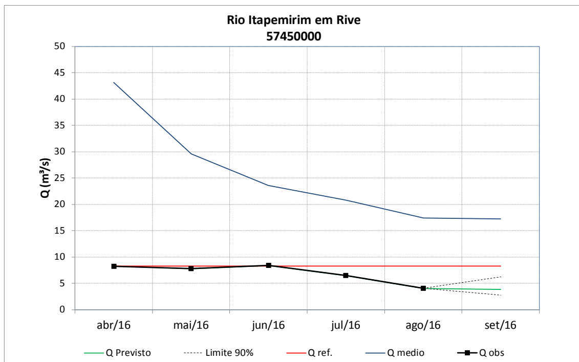
Figura 82 – Previsão de vazões médias do rio Itapemirim em Rive.
