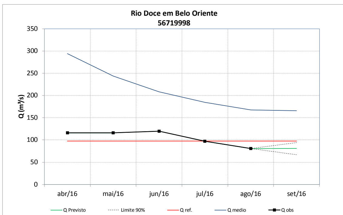
Figura 77 – Previsão de vazões médias do rio Doce em Belo Oriente.
