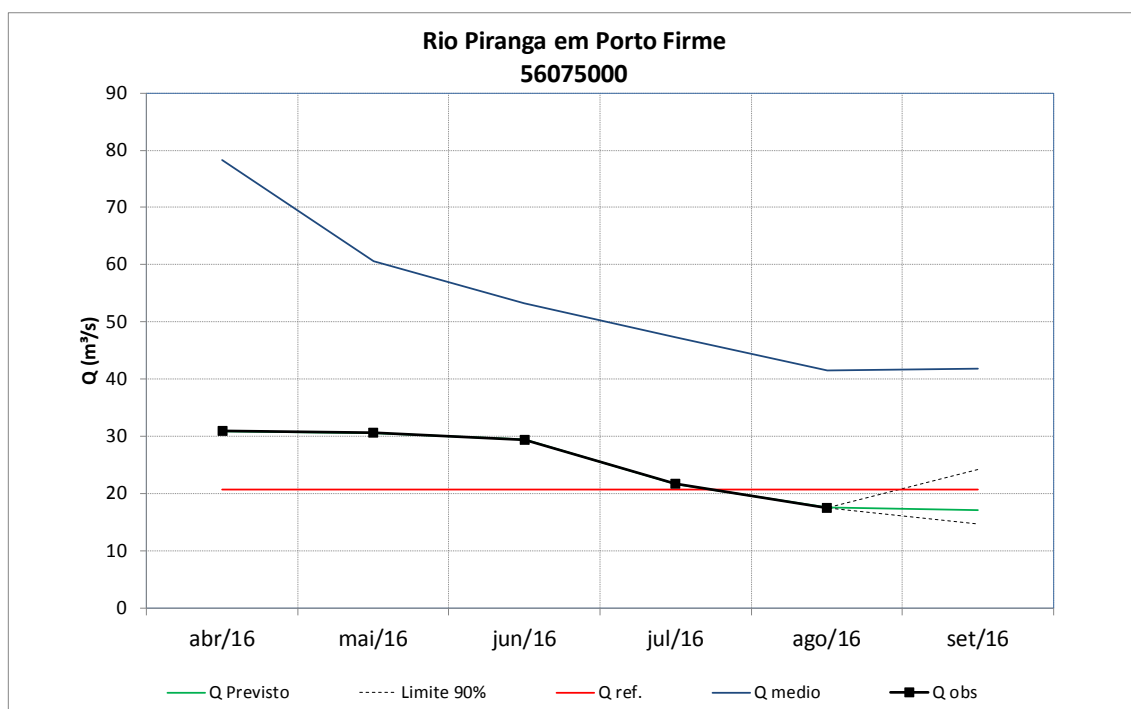
Figura 75 – Previsão de vazões médias do rio Piranga em Porto Firme.
