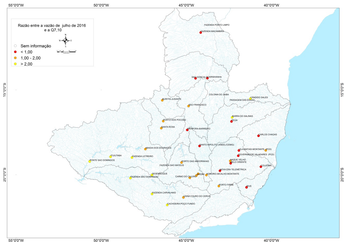
Figura 12 – Razão entre a vazão de julho de 2016 e a vazão Q 7,10 .
