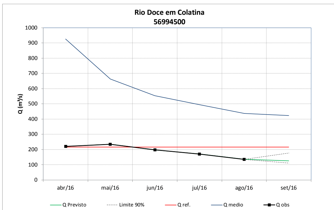
Figura 81 – Previsão de vazões médias do rio Doce em Colatina.
