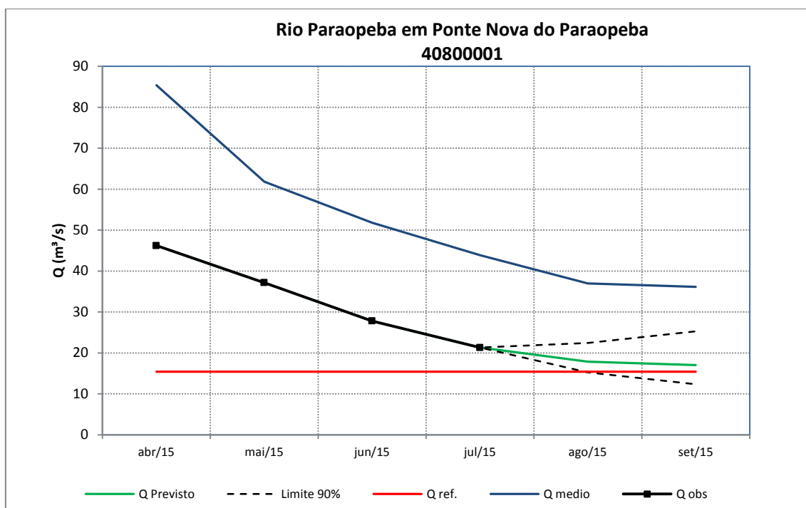
Figura 94 – Previsão de vazões médias do rio Paraopeba em Ponte Nova do Paraopeba
