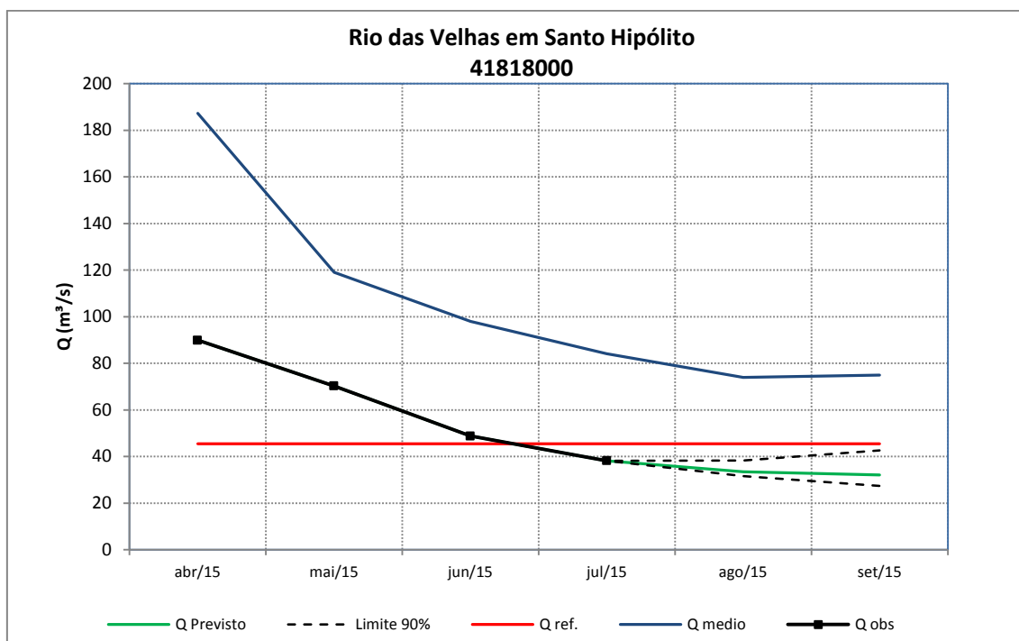
Figura 97 – Previsão de vazões médias mensais do rio das Velhas em Santo Hipólito.
