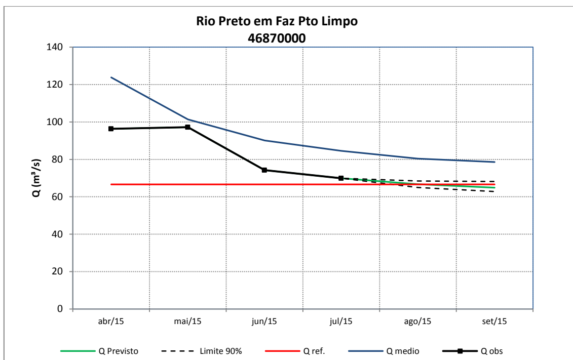
Figura 101 – Previsão de vazões médias mensais do rio Preto em Faz Pto Limpo.
