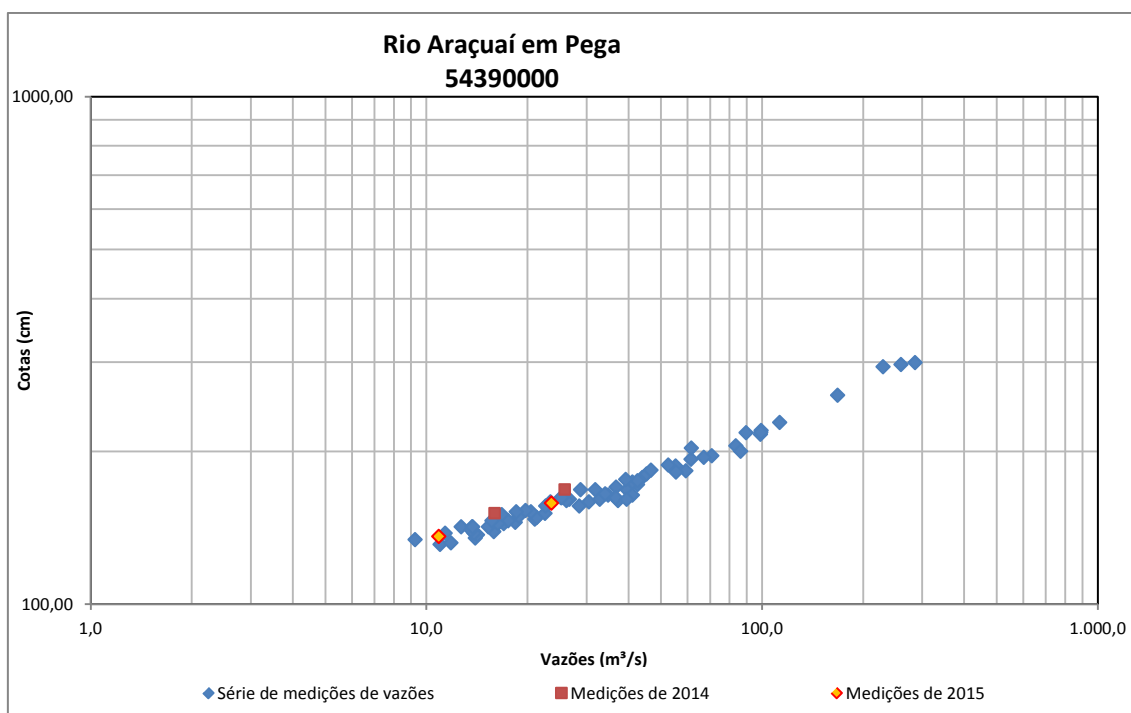
Figura 78 - Medições de descarga líquida do Rio Araçuaí em Pega
