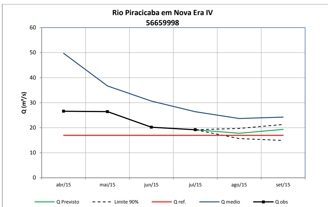
Figura 107 – Previsão de vazões médias mensais do rio Piracicaba em Nova Era IV.
