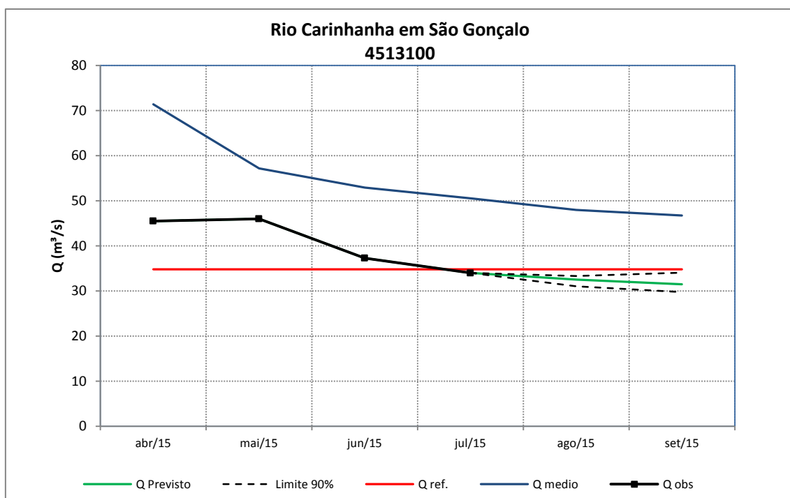
Figura 98 – Previsão de vazões médias mensais do rio Carinhanha em São Gonçalo.
