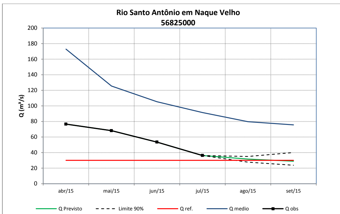
Figura 109 – Previsão de vazões médias mensais do rio Santo Antônio em Naque Velho.
