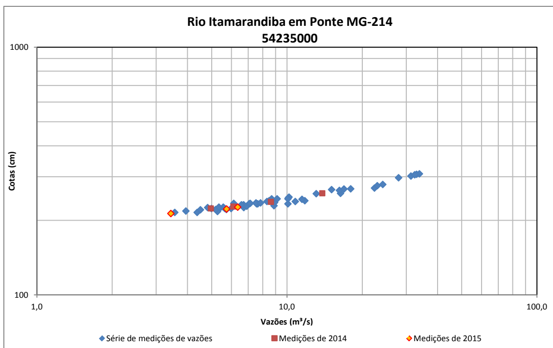
Figura 76 - Medições de descarga líquida do Rio Itamarandiba em Ponte MG-214
