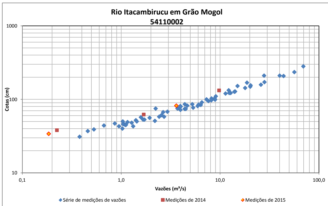
Figura 69 - Medições de descarga líquida do Rio Itacambirucu em Grão Mogol
