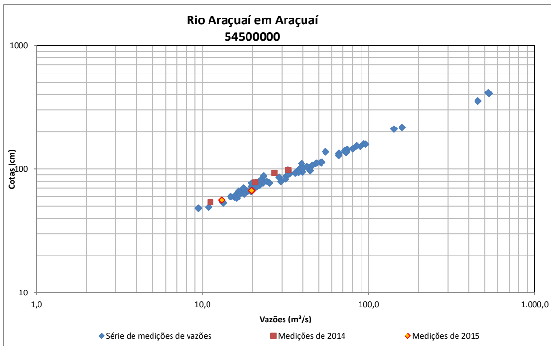
Figura 81 - Medições de descarga líquida do Rio Araçuaí em Araçuaí
