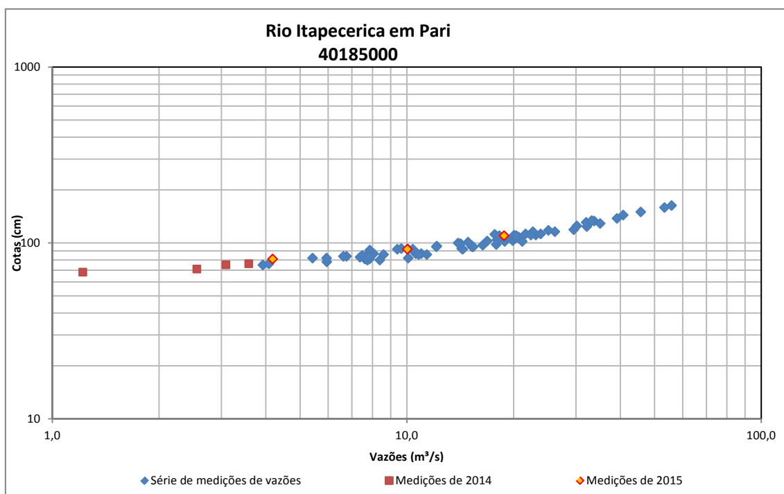
Figura 54 - Medições de descarga líquida do Rio Itapecerica em Pari
