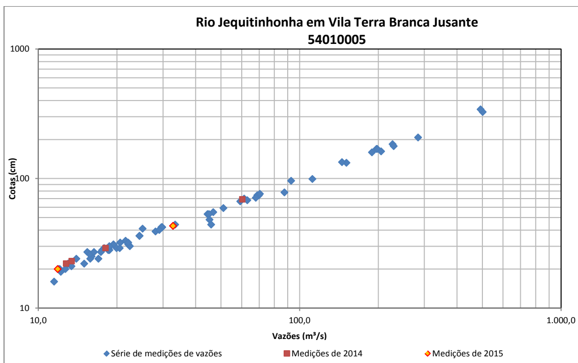
Figura 68 - Medições de descarga líquida do Rio Jequitinhonha em Vila Terra Branca Jusante
