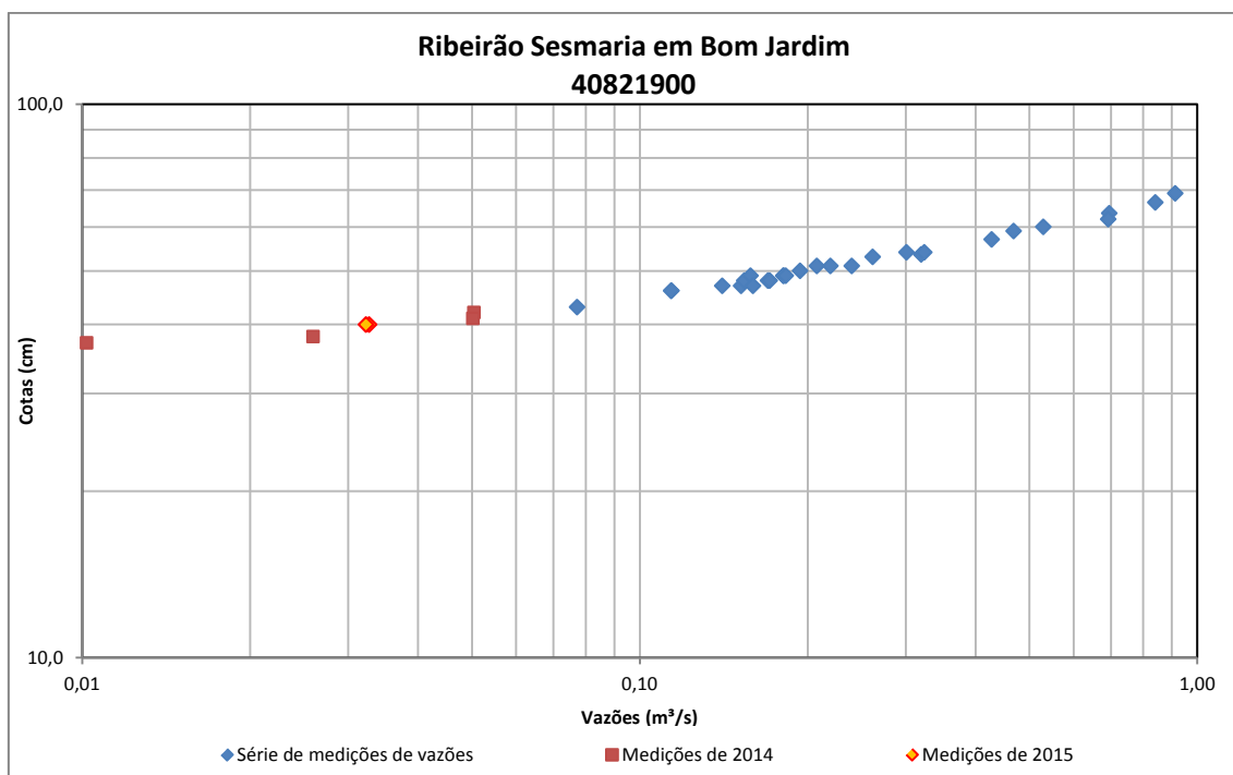
Figura 64 - Medições de descarga líquida do Ribeirão Sesmaria em Bom Jardim
