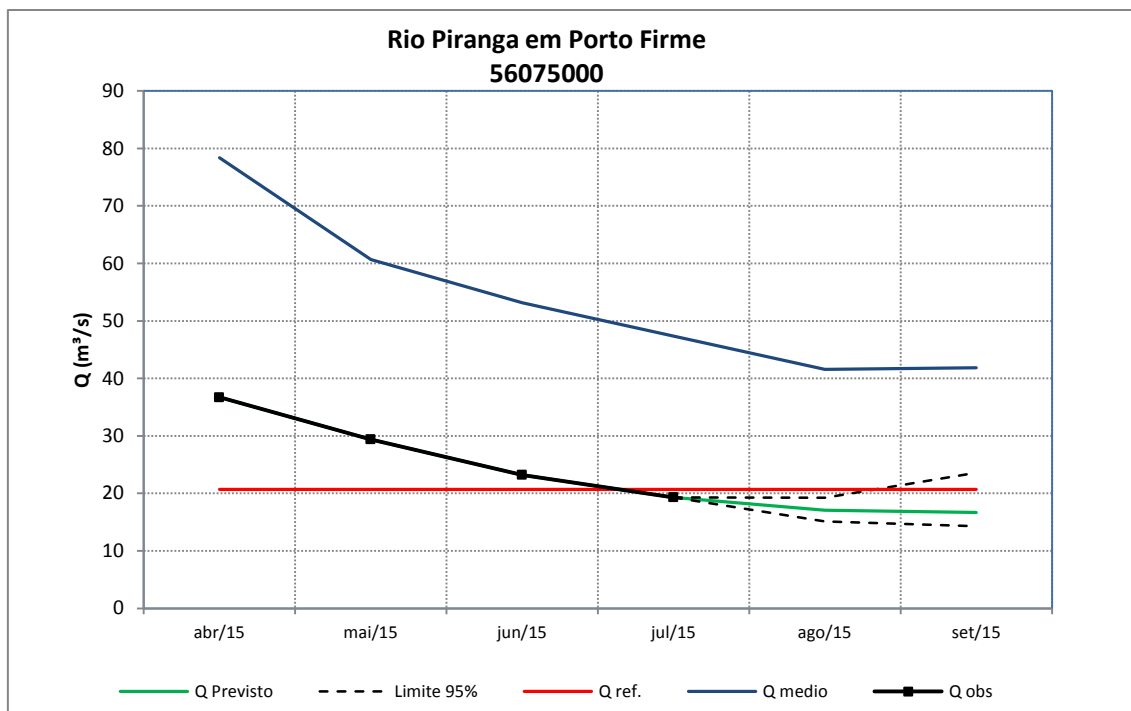
Figura 106 – Previsão de vazões médias mensais do rio Piranga em Porto Firme.
