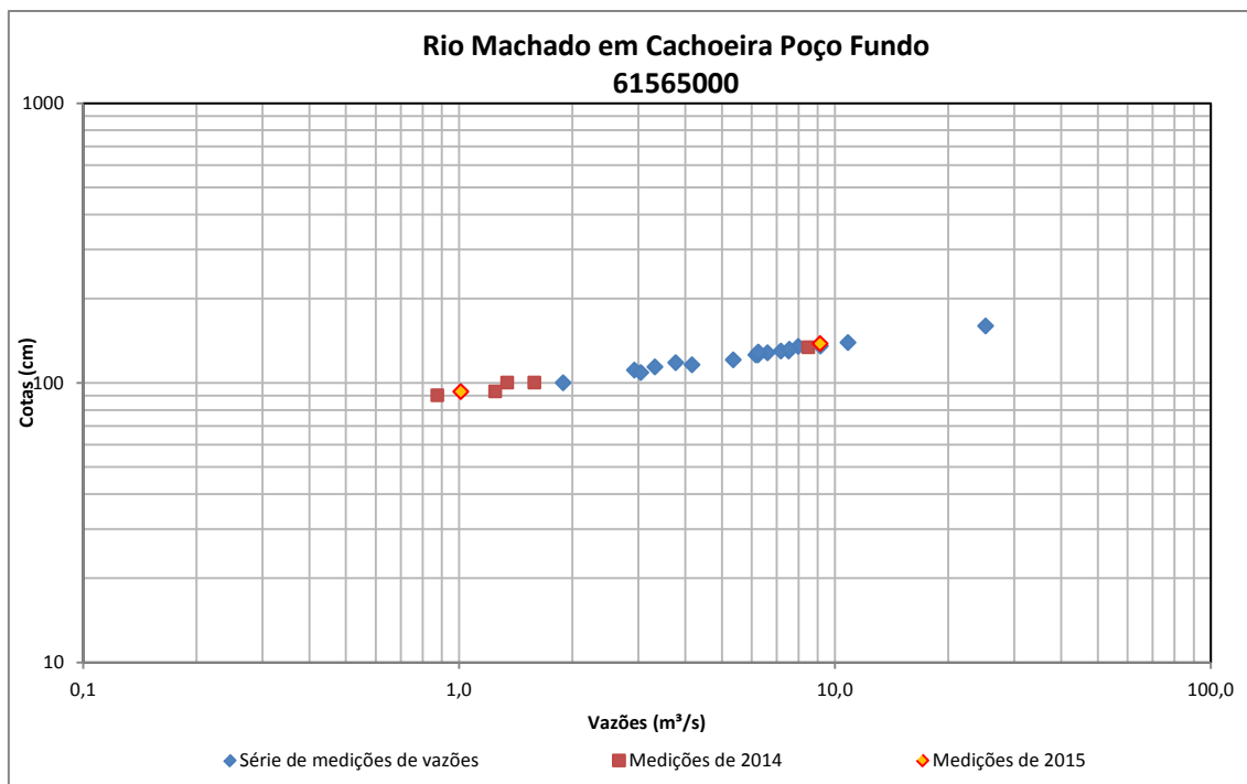
Figura 85 - Medições de descarga líquida do Rio Machado em Cachoeira Poço Fundo
