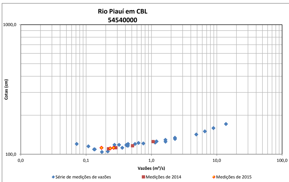
Figura 82 - Medições de descarga líquida do Rio Piauí em CBL
