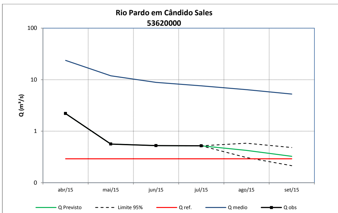
Figura 103 – Previsão de vazões médias mensais do rio Pardo em Cândido Sales.
