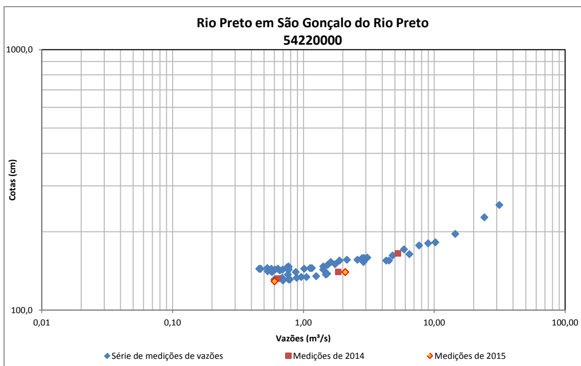
Figura 72 - Medições de descarga líquida do Rio Preto em São Gonçalo do Rio Preto
