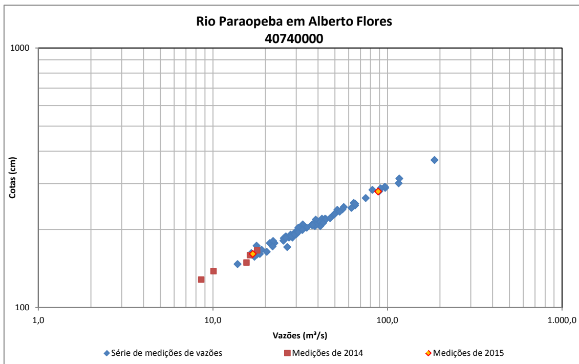
Figura 61 - Medições de descarga líquida do Rio Paraopeba em Alberto Flores
