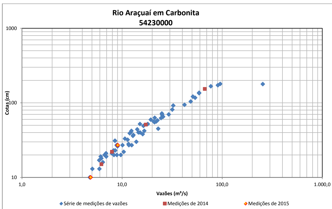
Figura 74 - Medições de descarga líquida do Rio Araçuaí em Carbonita
