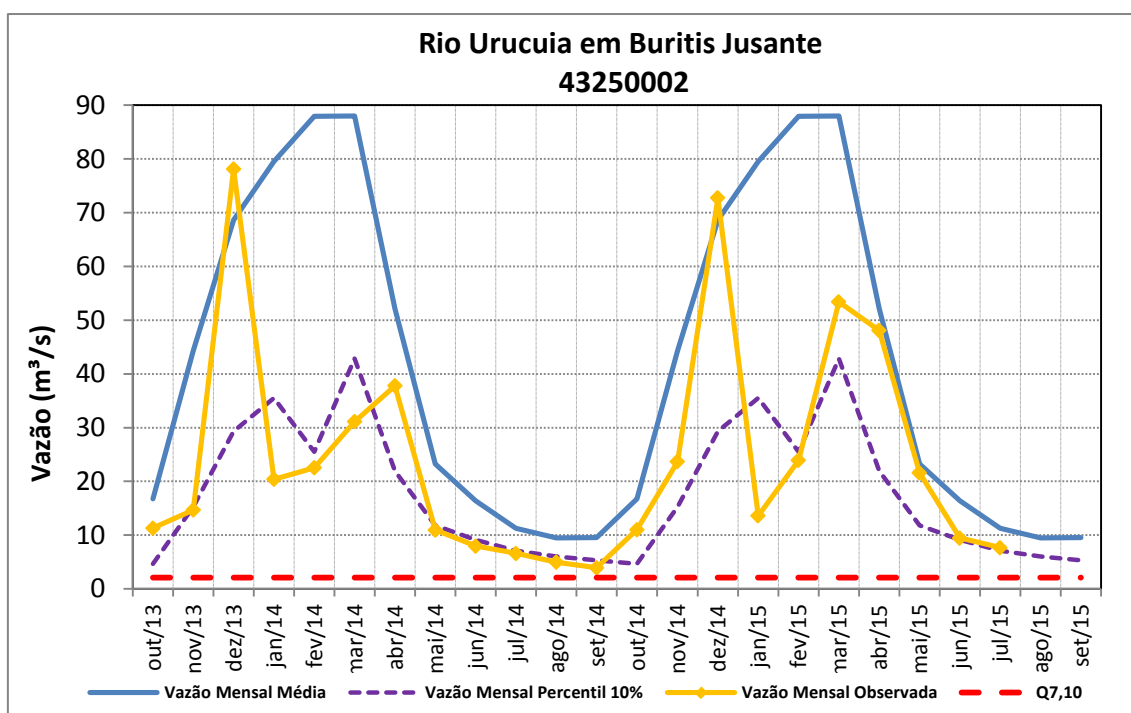
Figura 22 – Vazões médias mensais do rio Urucuia em Buritis Jusante.
