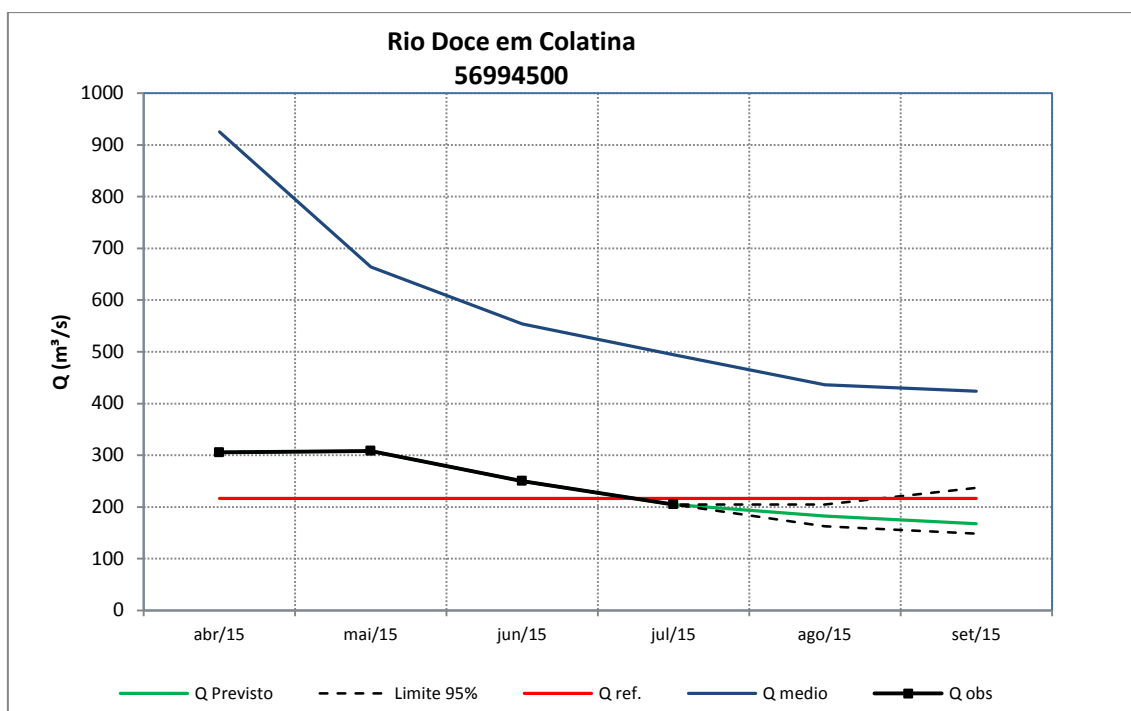
Figura 113 – Previsão de vazões médias mensais do rio Doce em Colatina.
