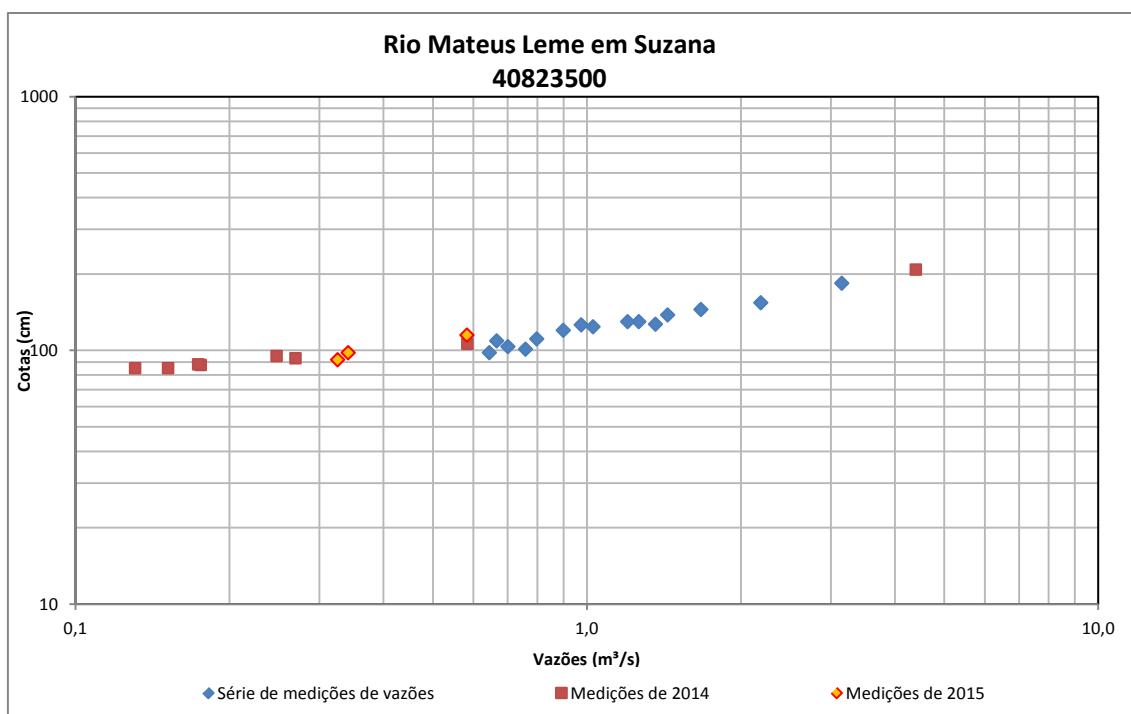
Figura 65 - Medições de descarga líquida do Rio Mateus Leme em Suzana
