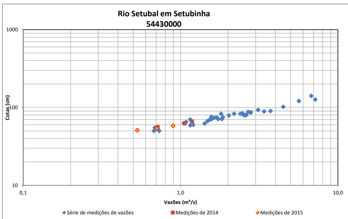
Figura 79 - Medições de descarga líquida do Rio Setubal em Setubinha
