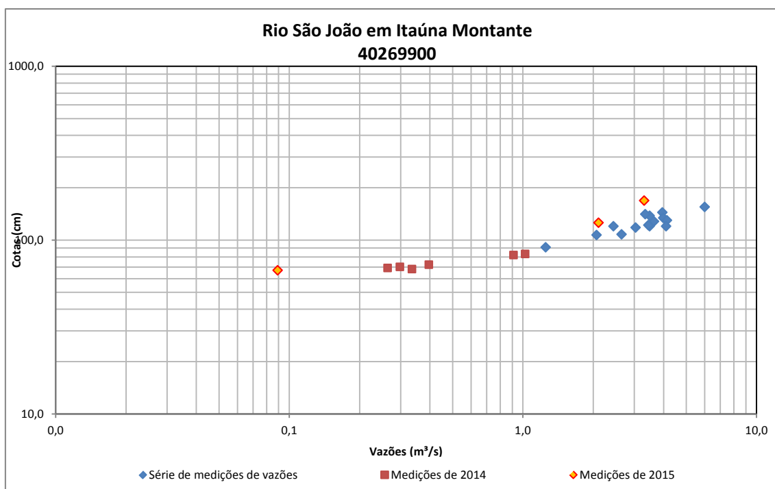
Figura 55 - Medições de descarga líquida do Rio São João em Itaúna Montante
