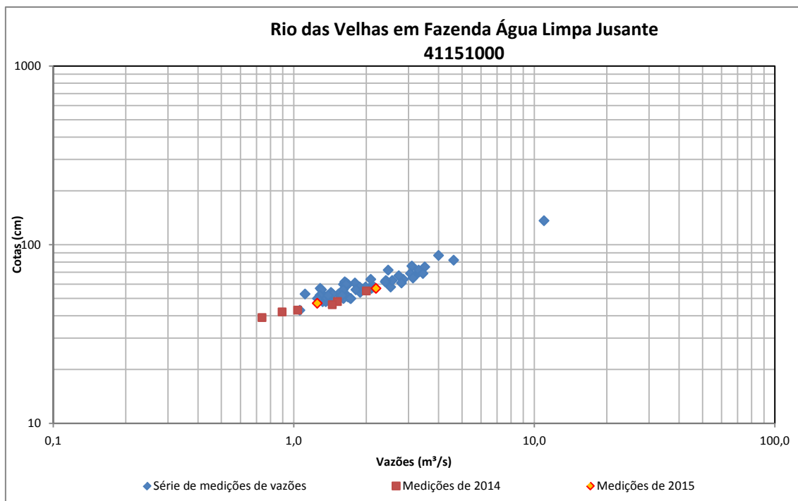
Figura 67 - Medições de descarga líquida do Rio das Velhas em Fazenda Água Limpa Jusante
