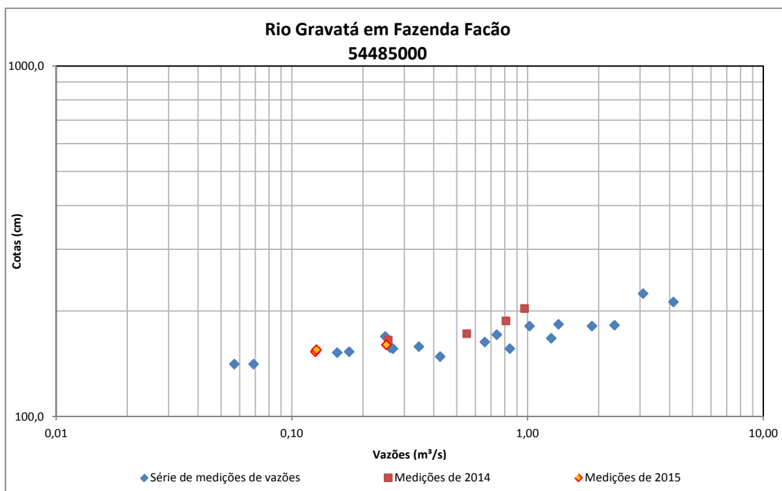
Figura 80 - Medições de descarga líquida do Rio Gravatá em Fazenda Facão
