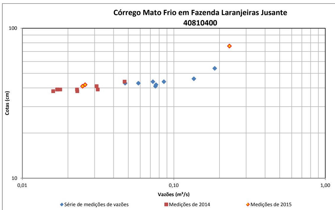
Figura 62 - Medições de descarga líquida do Córrego Mato Frio em Fazenda Laranjeiras Jusante
