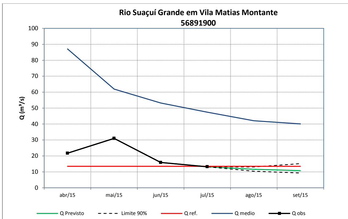
Figura 111 – Previsão de vazões médias mensais do rio Suaçuí Grande em Vila Matias Montante.
