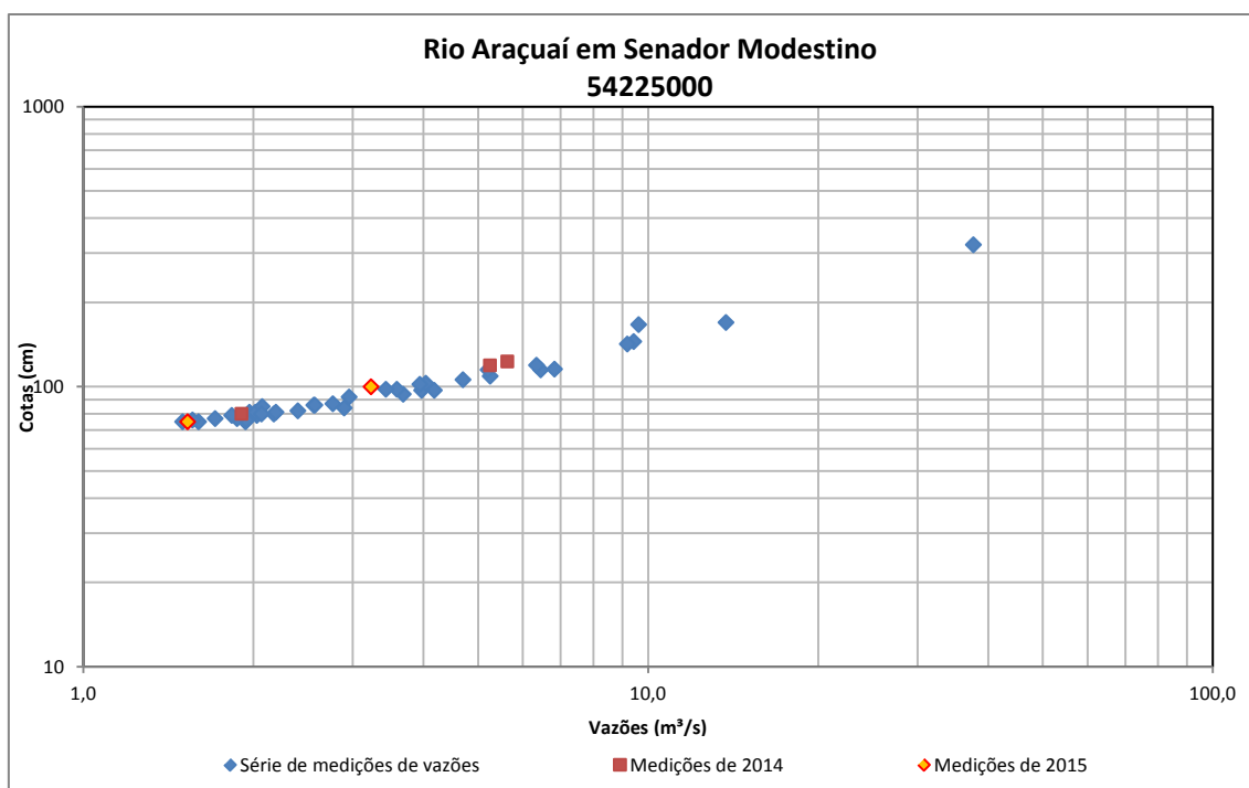
Figura 73 - Medições de descarga líquida do Rio Araçuaí em Senador Modestino
