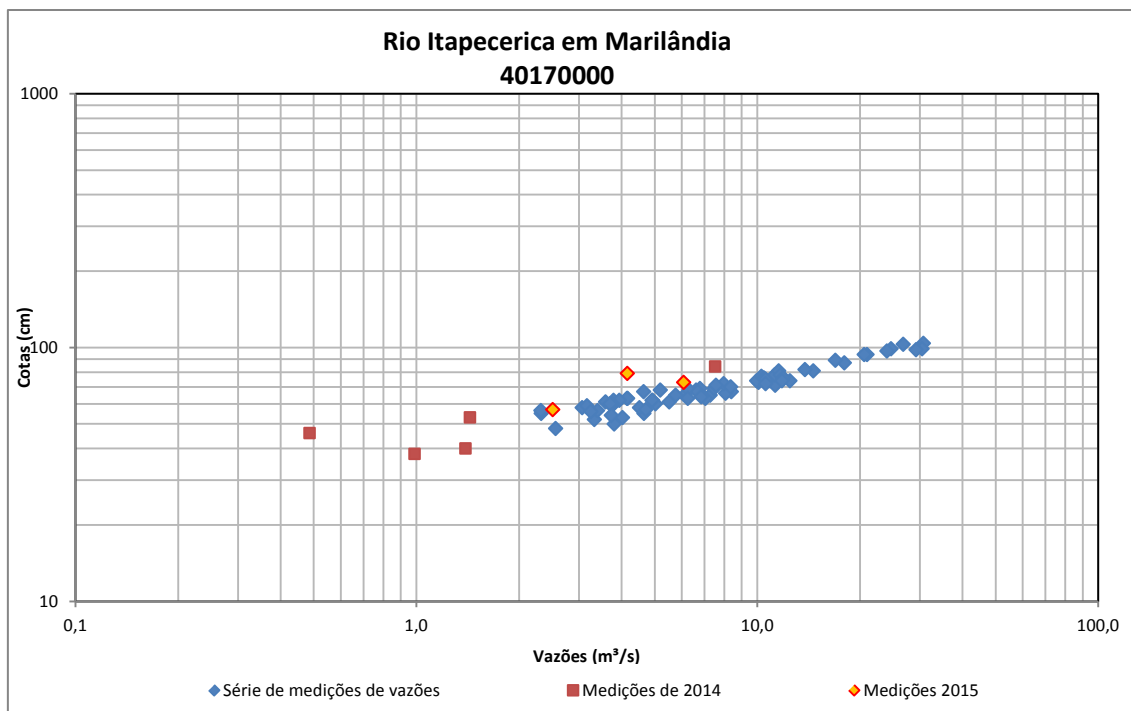
Figura 53 - Medições de descarga líquida do Rio Itapecerica em Marilândia
