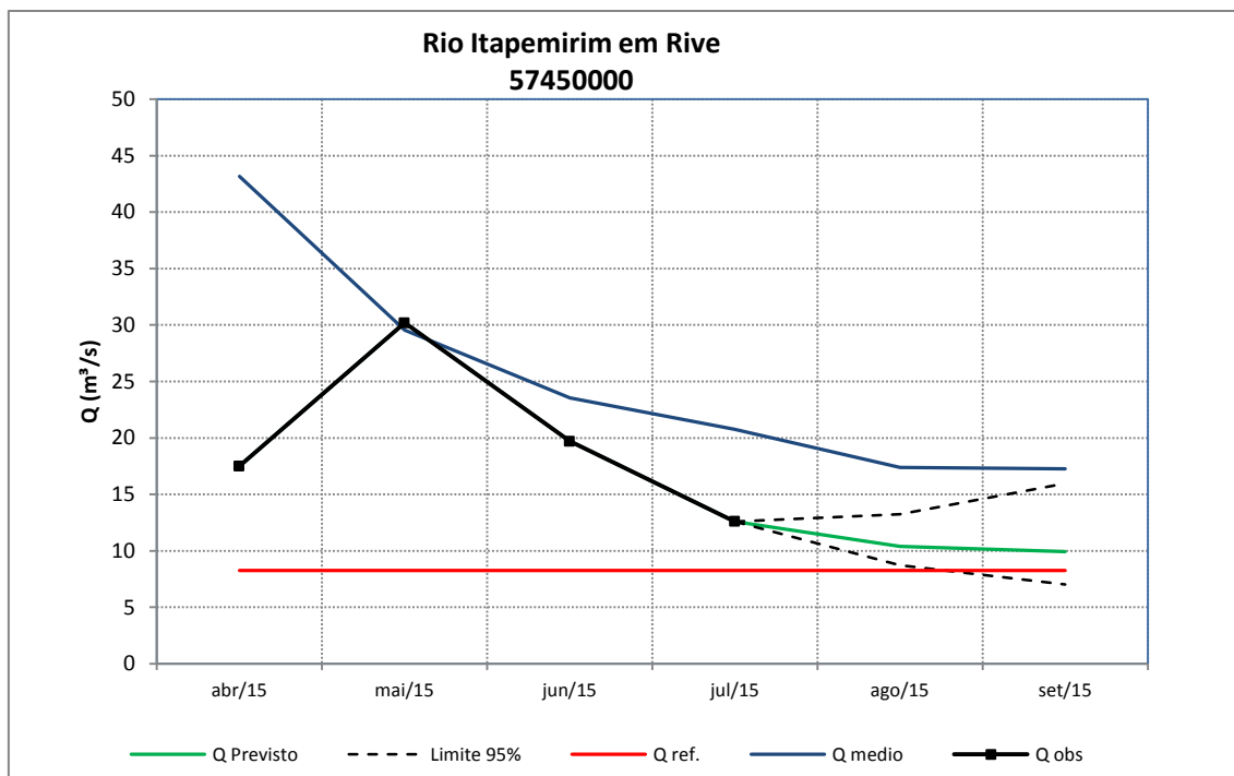
Figura 112 – Previsão de vazões médias mensais do rio Itapemirim em Rive.
