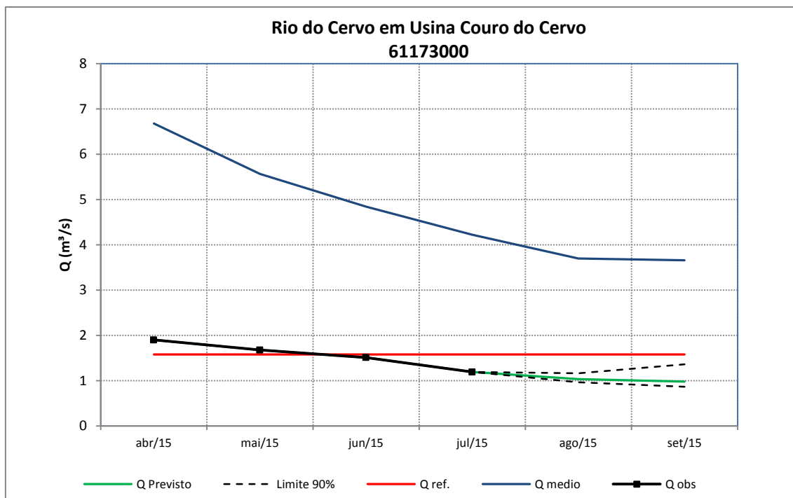
Figura 114 – Previsão de vazões médias mensais do rio do Cervo em Usina Couro do Cervo.
