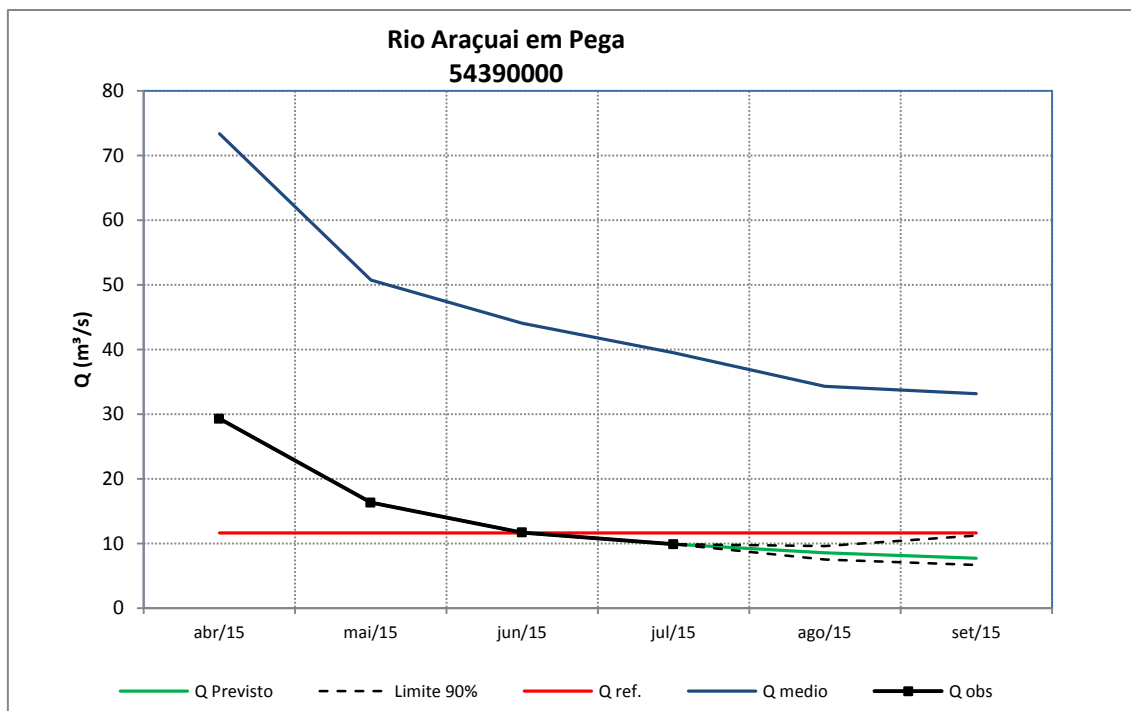
Figura 104 – Previsão de vazões médias mensais do rio Araçuaí em Pega.
