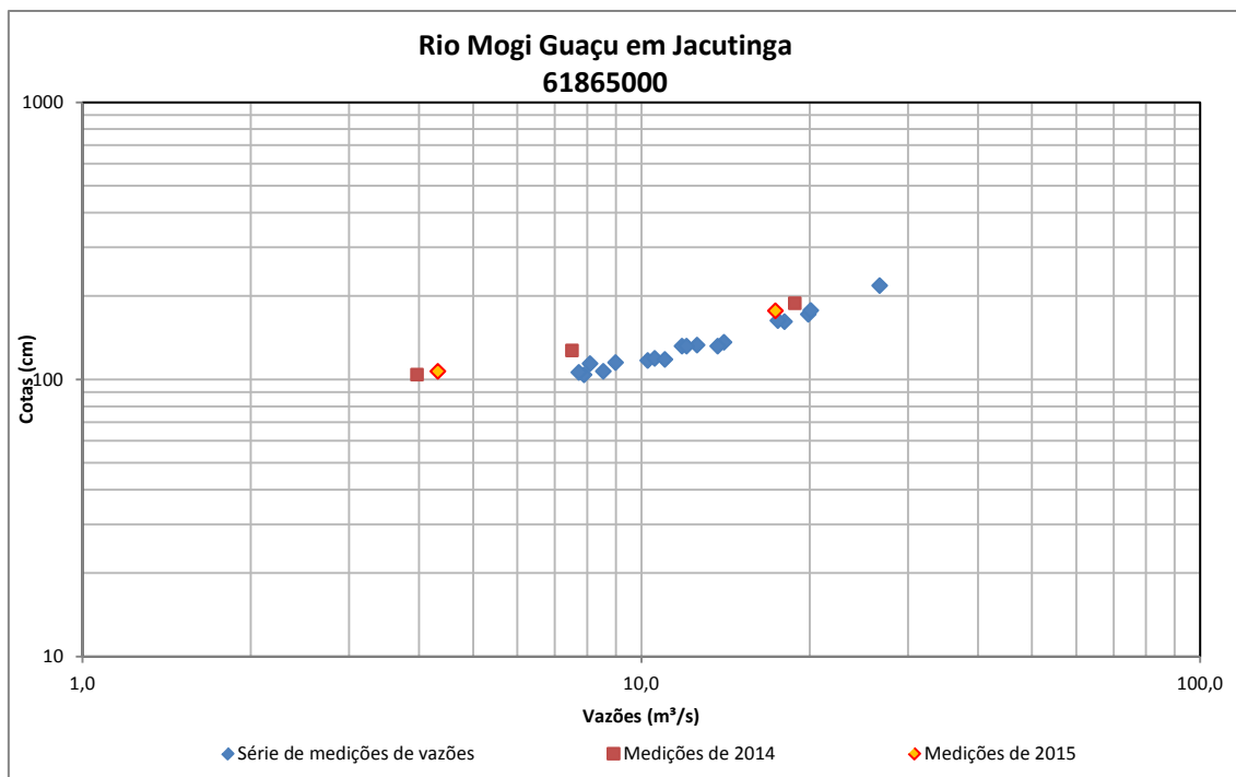
Figura 93 - Medições de descarga líquida do Rio Mogi Guaçu em Jacutinga
