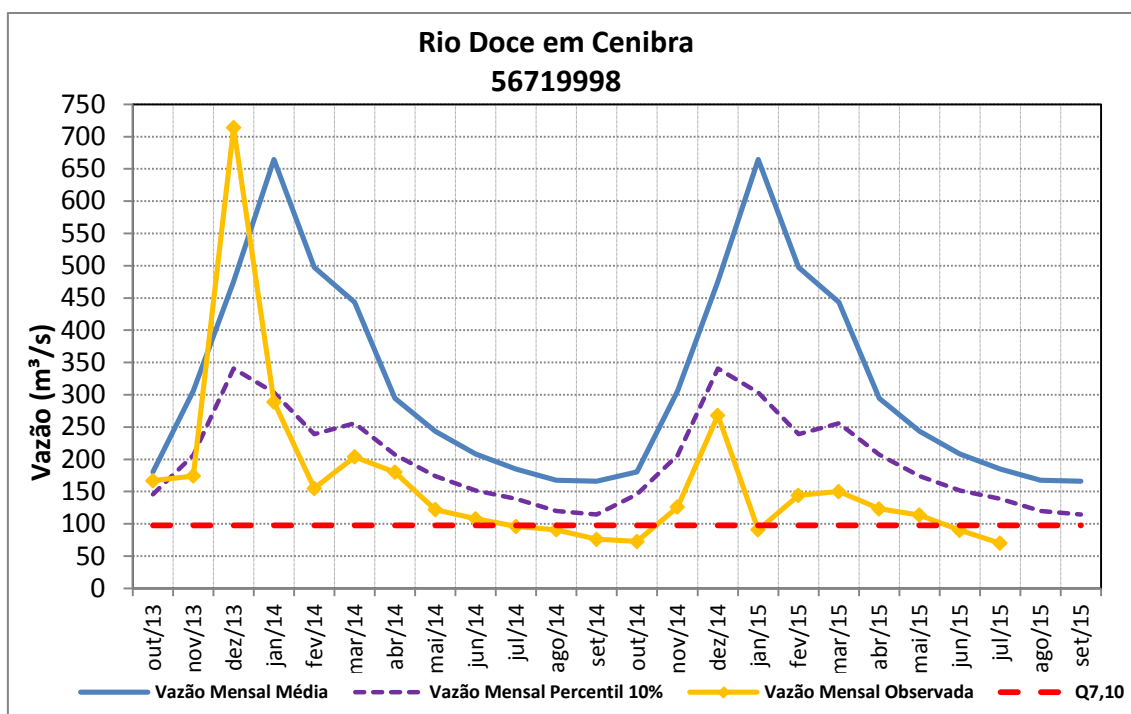
Figura 37 – Vazões médias mensais do rio Doce em Cenibra.
