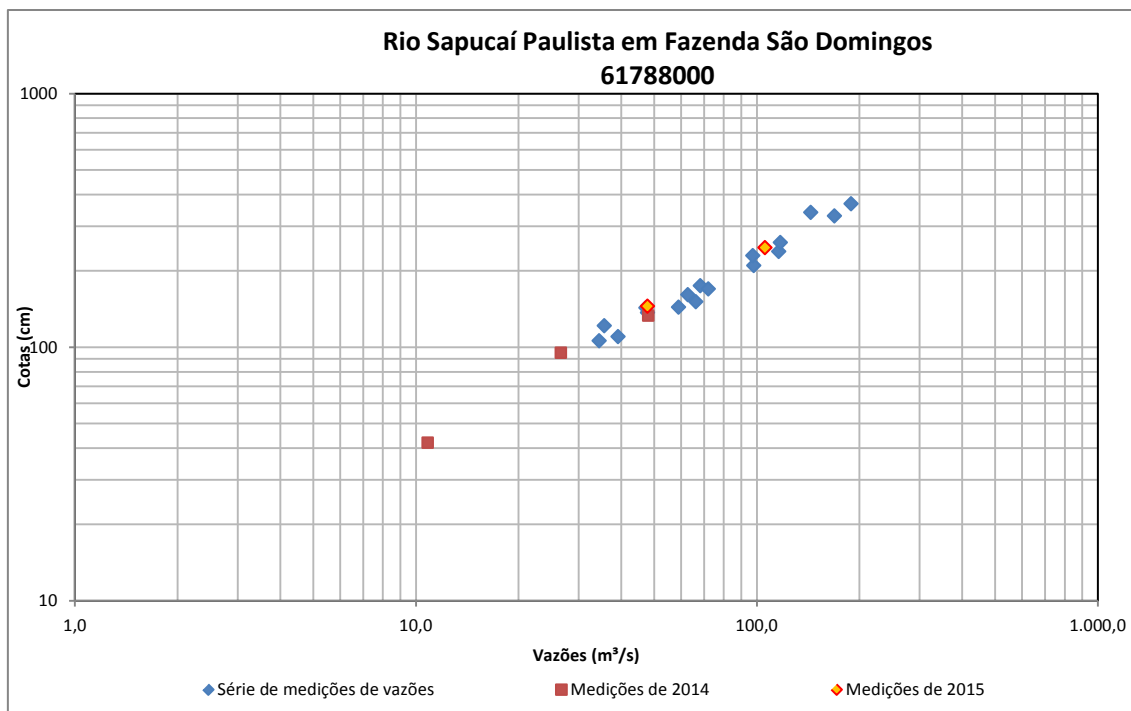
Figura 89 - Medições de descarga líquida do Rio Sapucaí Paulista em Fazenda São Domingos
