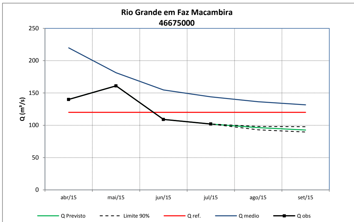
Figura 100 – Previsão de vazões médias mensais do rio Grande em Fazenda Macambira.
