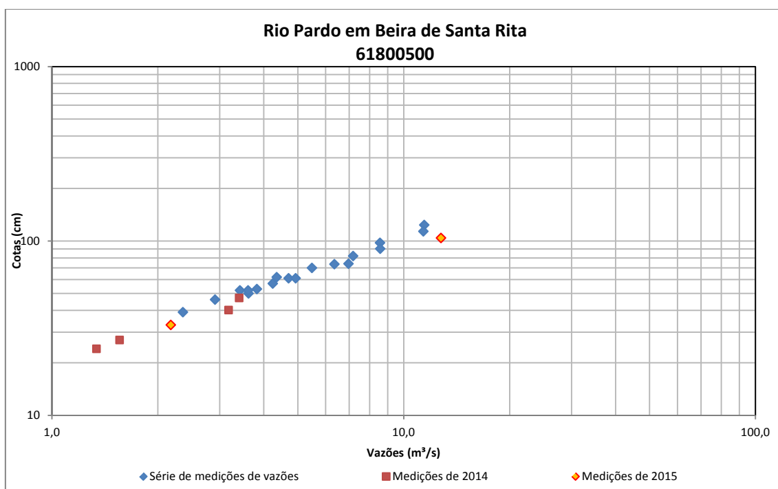
Figura 90 - Medições de descarga líquida do Rio Pardo em Beira de Santa Rita
