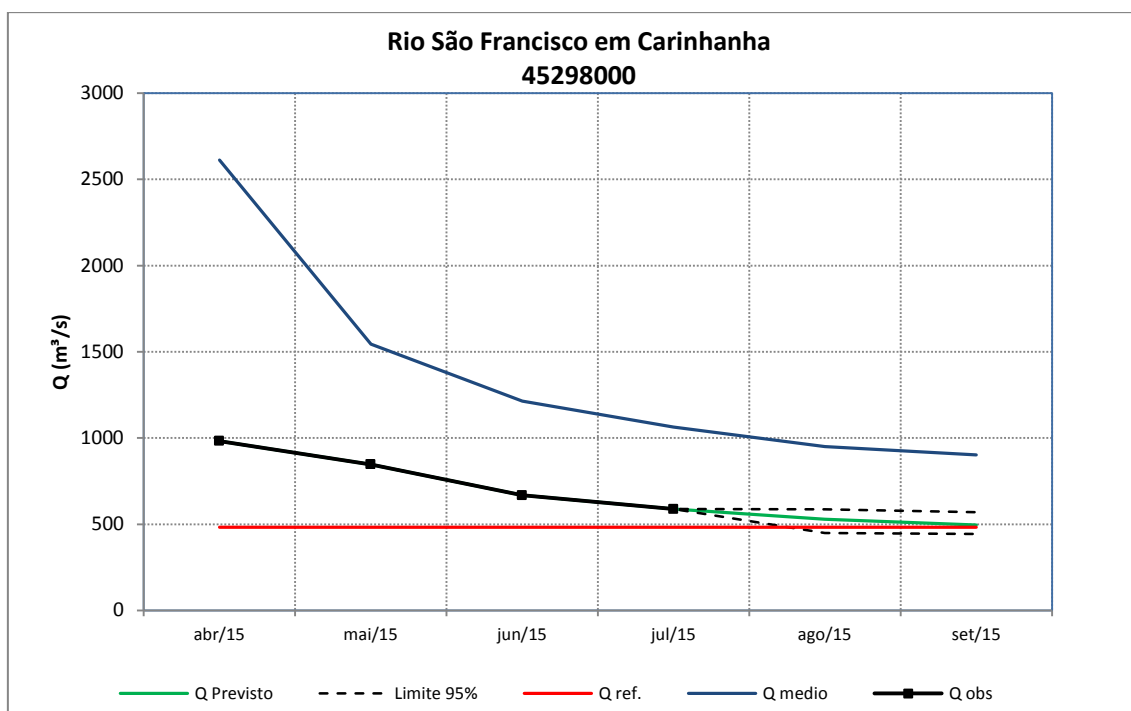
Figura 99 – Previsão de vazões médias mensais do rio São Francisco em Carinhanha.
