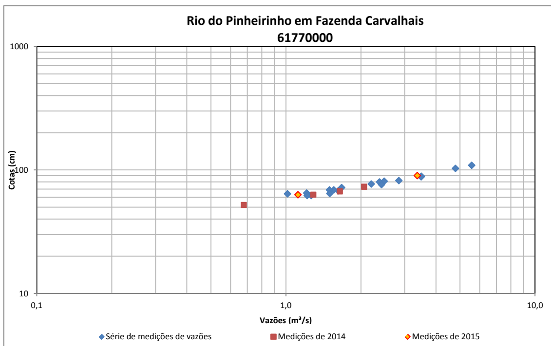
Figura 88 - Medições de descarga líquida do Rio do Pinheirinho em Fazenda Carvalhais
