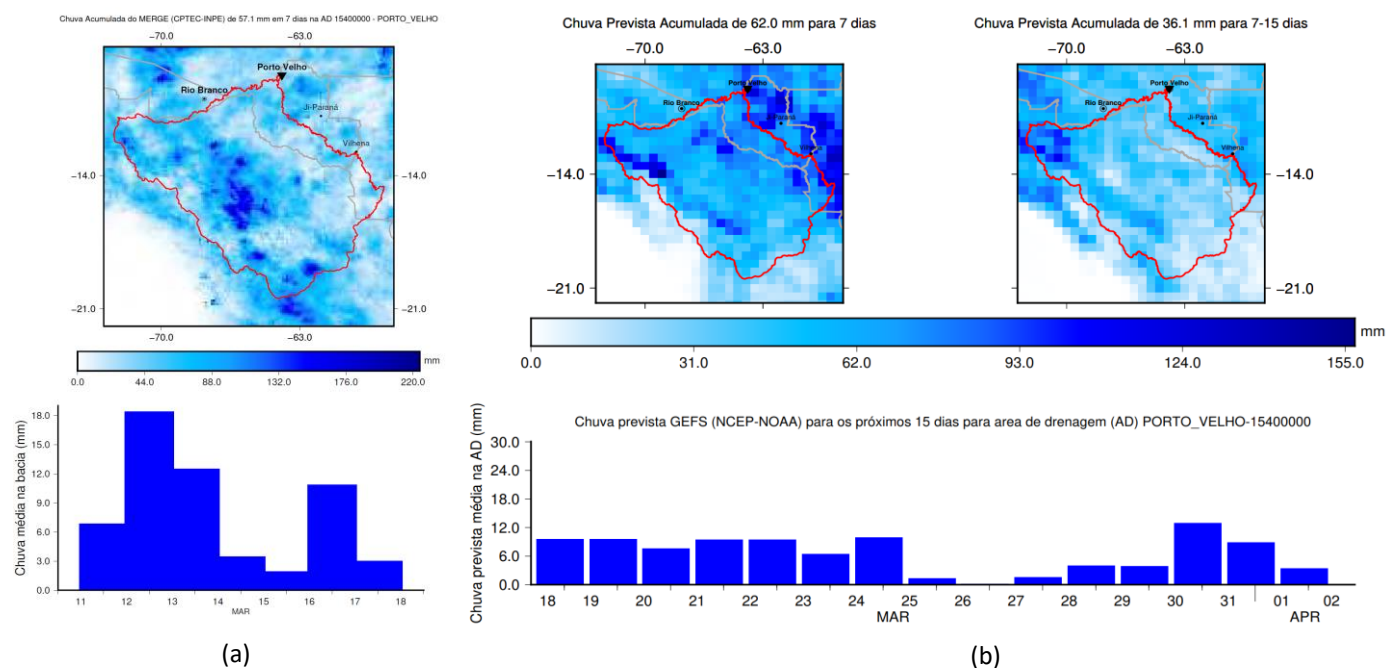
Figura 3. Chuvas observadas ao longo da última semana na bacia do Rio Madeira (57 mm), delimitada à jusante pela estação de Porto Velho (a); média da previsão de 20 membros do Ensemble do GEFS/NOAA (62 mm e 36 mm na primeira e segunda semanas, respectivamente).
