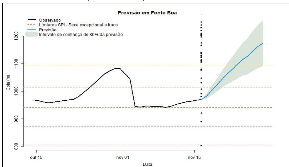
Figura 15: previsão para rio Solimões em Fonte Boa, utilizando modelo Cota-cota, utilizando a previsão de precipitação por ensemble a partir do modelo GEFS.
