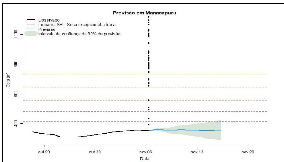
Figura 10: previsão para rio Solimões em Manacapuru, utilizando modelo Cota-cota, utilizando a previsão de precipitação por ensemble a partir do modelo GEFS.
