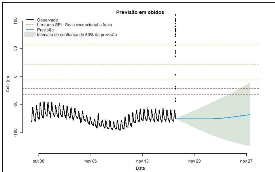
Figura 14: previsão para rio Amazonas em Óbidos, utilizando modelo Cota-cota, utilizando a previsão de precipitação por ensemble a partir do modelo GEFS.
