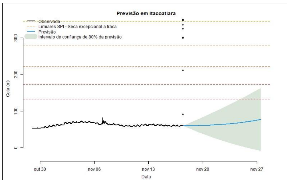
Figura 12: previsão para rio Amazonas em Itacoatiara, utilizando modelo Cota-cota, utilizando a previsão de precipitação por ensemble a partir do modelo GEFS.
