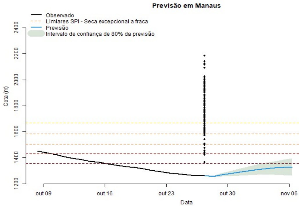
Figura 09: previsão para rio Negro em Manaus, utilizando modelo Cota-cota, utilizando a previsão de precipitação por ensemble a partir do modelo GEFS.
