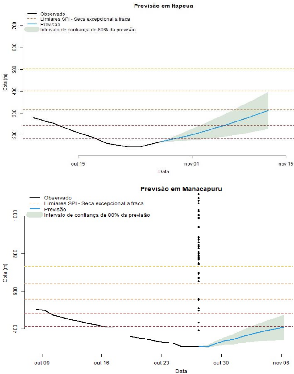
Figura 08: previsão para rio Solimões em Itapeua e Manacapuru, utilizando modelo Cota-cota, utilizando a previsão de precipitação por ensemble a partir do modelo GEFS.
