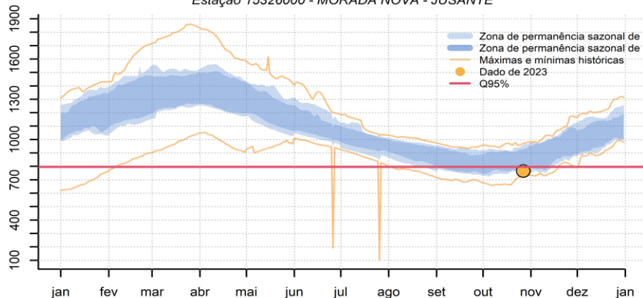
Histórico de registro de níveis e comparativo com dado de 2023 Estação 15326000 - MORADA NOVA - JUSANTE
