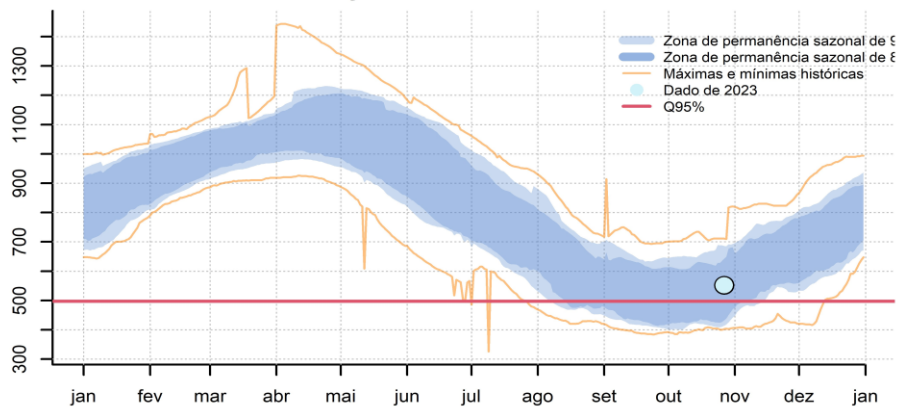
Histórico de registro de níveis e comparativo com dado de 2023 Estação 15250000 - GUAJARA-MIRIM
