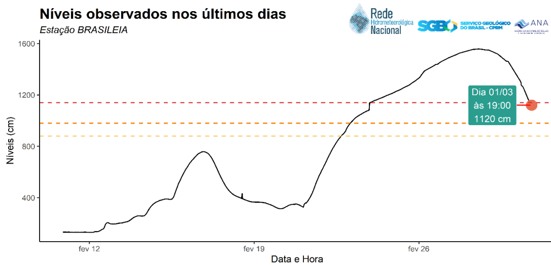
Figura 3. Níveis do rio Acre na estação de Brasília no município de Brasília-AC nas últimas 2 semanas
