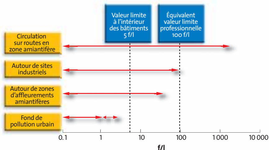
▲ Fig. 1 : Niveaux potentiels d'exposition aux fibres d'amiante mesurés en France dans différents environnements. Fig. 1: Potential levels of exposure to asbestos fibres in France in various environments.
