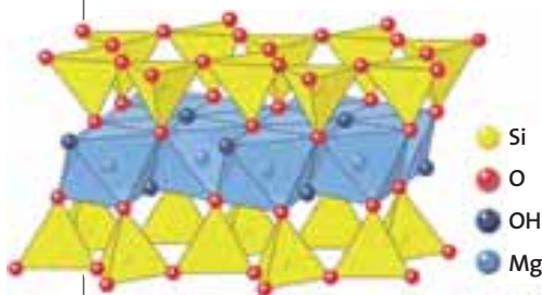
▲ Feuillet élémentaire de talc. An elementary sheet of talc.
