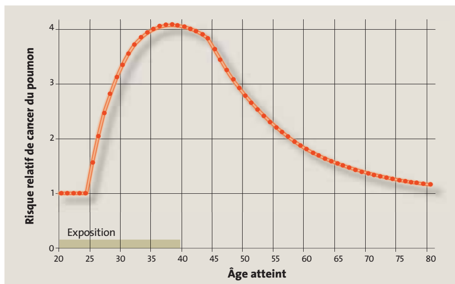
Fig. 1 : Scénario réalisé d'après les résultats du suivi des mineurs d'uranium ; études menées dans le cadre des 5 ème et 6 ème PCRD (programme de recherche européen « alpha-risk »). Il s'agit du cas d'un mineur exposé à partir de l'âge de 20 ans à 2 WLM (unité d'exposition « mine » équivalente à 460 Bq par m 3 dans l'habitat) par an pendant 20 ans. Le risque commence à augmenter après un temps de latence de 5 ans, atteint un maximum à l'âge de 40 ans, puis commence à diminuer au fur et à mesure que l'on s'éloigne de la période d'exposition.
