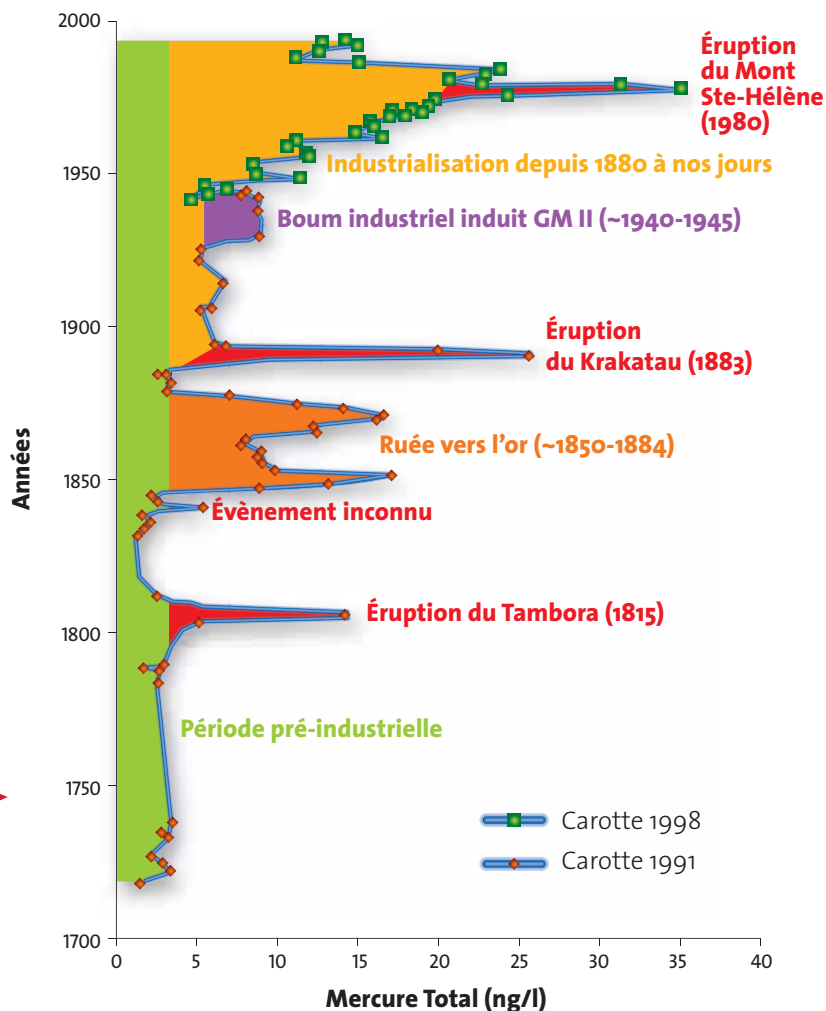
Fig. 1 : Données sur la distribution du mercure enregistré dans les glaces polaires. La partie verte correspond au fond naturel en mercure extrapolée à partir des données les plus anciennes ; les parties rouges aux contributions volcaniques majeures (Krabbenhoft et Schuster, 2002).
