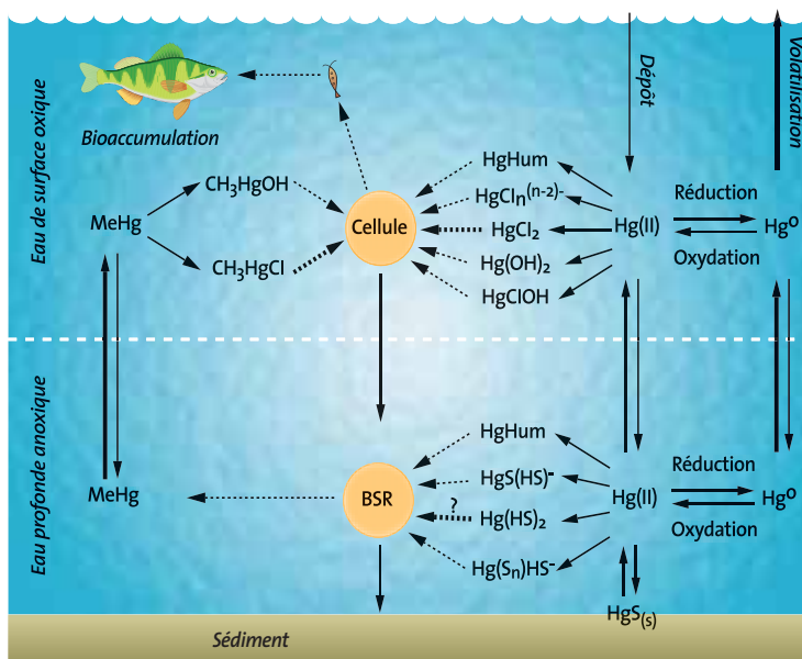
▲ Cycle du mercure dans l'hydrosphère. BSR : Bactéries Sulfato-Réductrices. Mercury cycle in the hydrosphere. BSR (Bactéries Sulfato-Réductrices): sulphate-reducing bacteria.
